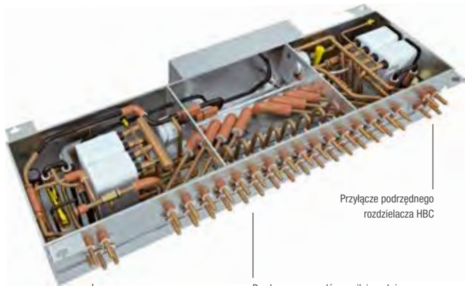
Przylącza przewodów zasilających i powrotnych do systemu wodociągowego; dostępne są wersje z 8 lub 16 przylącami.
